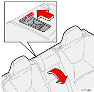
Rückenlehne des mittleren Sitzplatzes (XC70 mit dreigeteilter Rücksitzbank)
