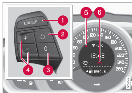
Tastenfeld des Lenkrads und Display in einem Fahrzeug ohne Geschwindigkeitsbegrenzung 6 .
