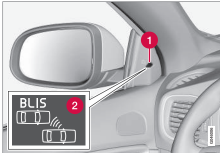
Platzierung der BLIS-Leuchte 32 .
