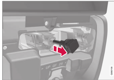
Lampengehäuse links.
