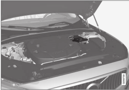
Die Unterstützungsbatterie befindet sich in einem Gehäuse neben dem Federbeinturm.
