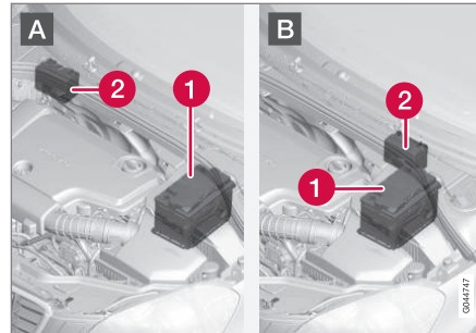
A: Linksenker. B: Rechtslenker. (1) Startbatterie 12 (2) Unterstützungsbatterie.
