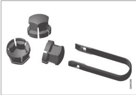
Ausbauwerkzeug für die Kunststoffkappen der Radmuttern.
