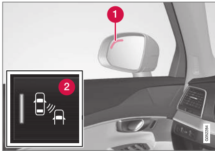
Lage der BLIS-Leuchte 88 .
