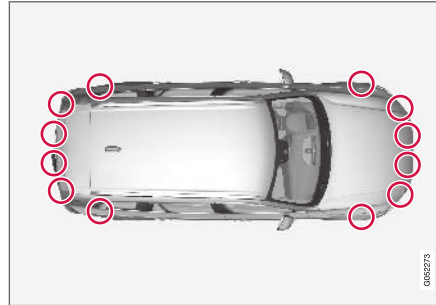
Lage der Einparkhilfesensoren 126 .
