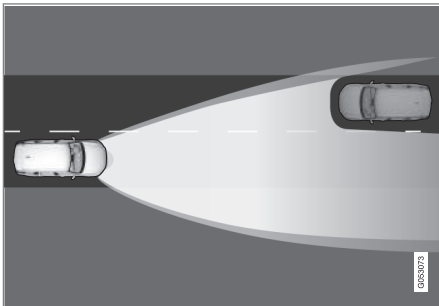
Adaptive Funktion: Abblendet direkt in Richtung entgegenkommender Fahrzeuge, aber weiterhin Fernlicht auf beiden Seiten des Fahrzeugs.
