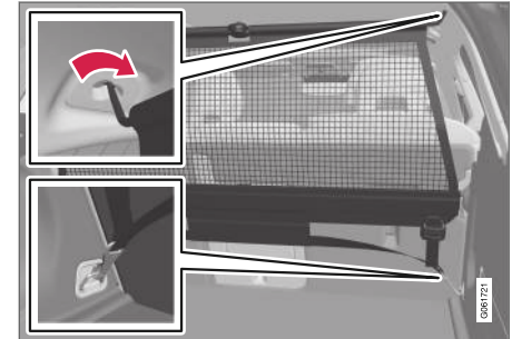
Montage hinten.
