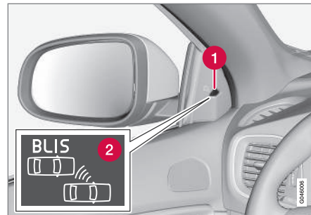
Platzierung der BLIS-Leuchte 38 .
