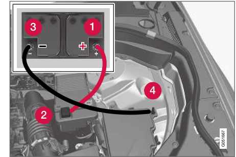
Anschlusspunkte der Starthilfekabel.
