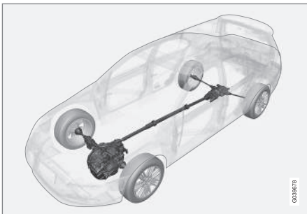
AWD-Prinzip 9 .
