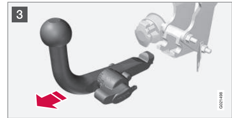
3 Den Verriegelungsknopf vollständig bis zum Anschlag weiterdrehen, herunterdrücken und gleichzeitig die Anhängierzugvorrichtung nach hinten und oben herausziehen.
