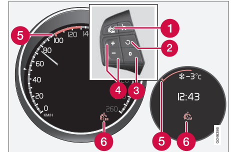
Tastenfeld des Lenkrads und Kombinationsinstrument Digital bzw. Analog.
