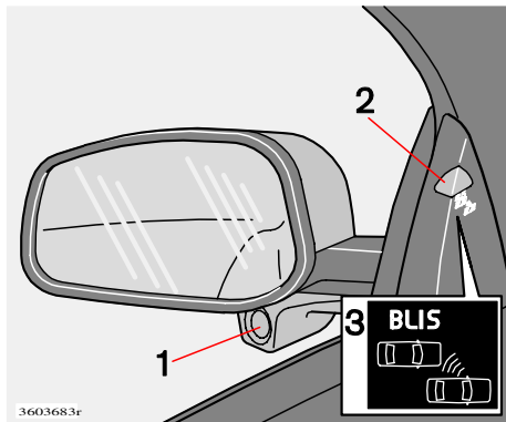
1 - BLIS-Kamera, 2 - Anzeigeleuchte, 3 - BLIS-Symbol
