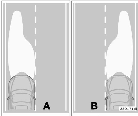
A. Lichtmuster für Linksverkehr B. Lichtmuster für Rechtsverkehr
