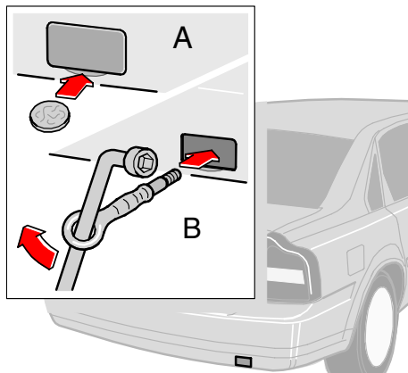
Abschleppöse, hinten
