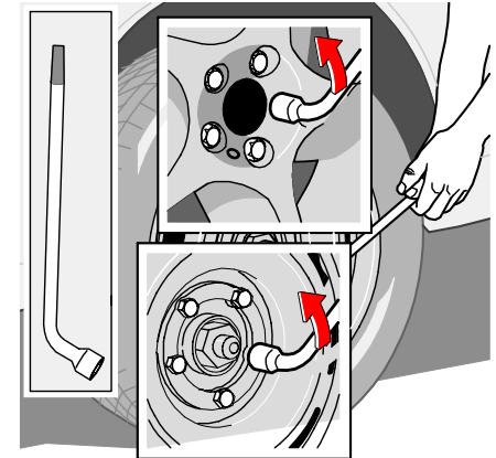
Radbolzen lösen
