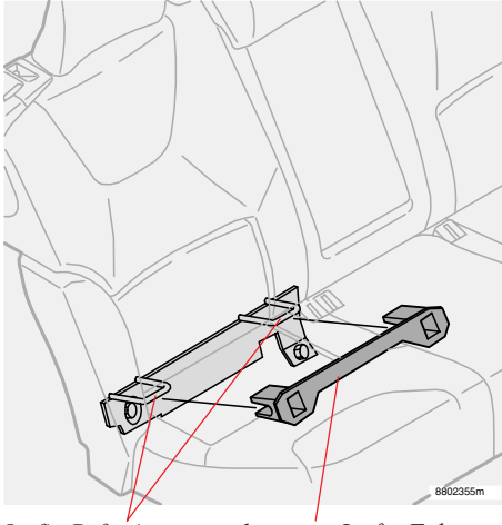
Isfix-Befestigungspunkte
