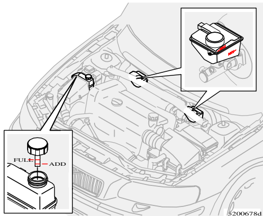
Servolenkölbehälter
