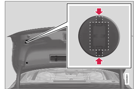
Die rechteckige Partie der Clips weist in Längsrichtung des Fahrzeugs.
