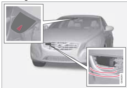
Kamera- und Radarsensor 3 .
