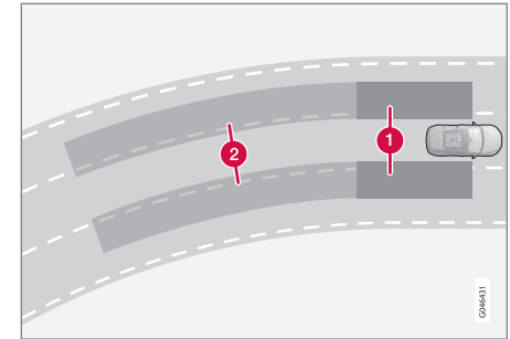
Prinzip für BLIS: 1. Zone im toten Winkel. 2. Zone für schnell aufholende Fahrzeuge.
