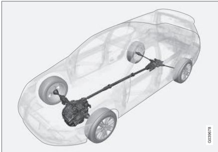
AWD-Prinzip 10 .
