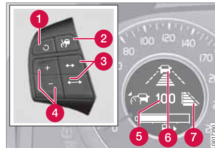
Tastenfeld des Lenkrads und Display in einem Fahrzeug ohne Geschwindigkeitsbegrenzer 3 .
