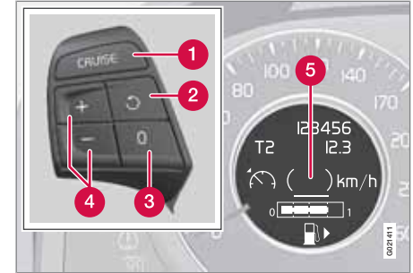
Tastenfeld des Lenkrads und Display in einem Fahrzeug ohne Geschwindigkeitsbegrenzer 1 .
