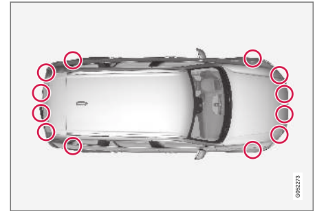
Lage der Einparkhilfesensoren 138 .
